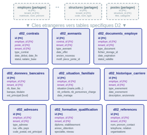
Figure 2.1 - Modele de donnees du Domaine D2 (Gestion Administrative du Personnel)
