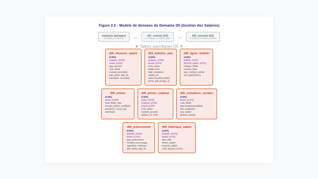
Figure 2.2 - Schema entite-association du domaine D5
