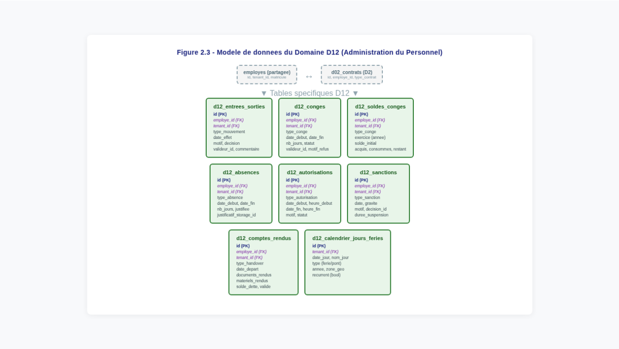
Figure 2.3 - Schema entite-association du domaine D12
